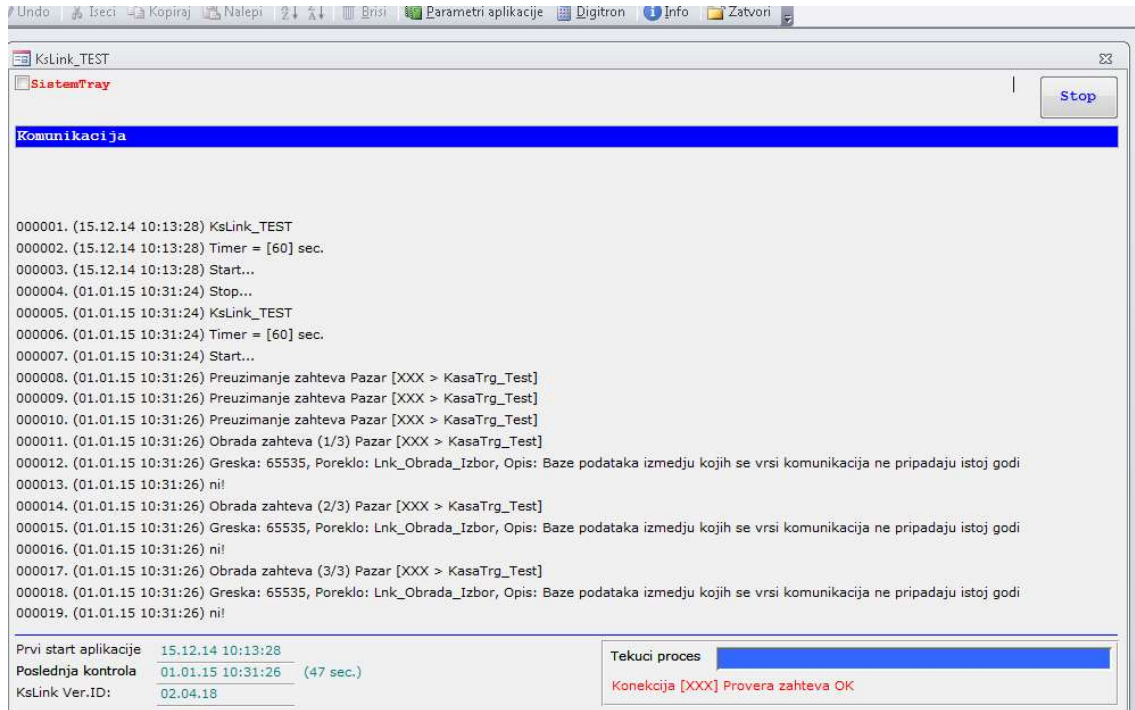
Slika 15 KLinkSQL
